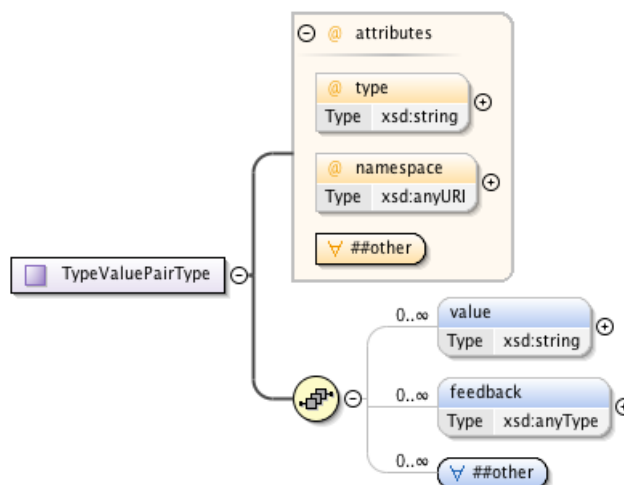
Figure 21 – TypeValuePairType type.
