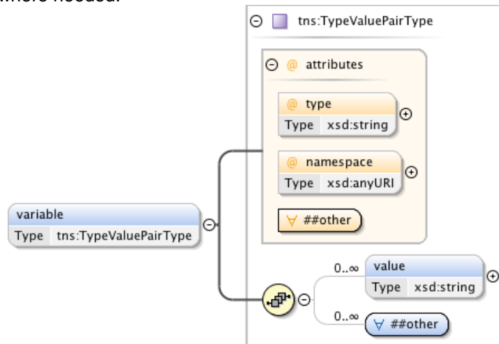
Figure 21 – TypeValuePairType type.
